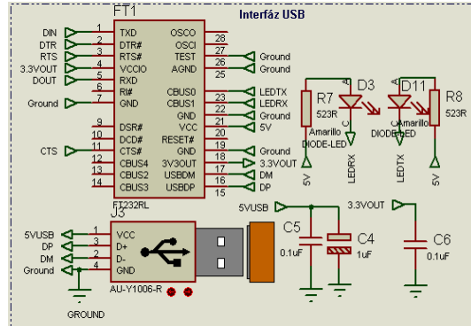
Figura 8. Interfaz serial USB 2.0.
