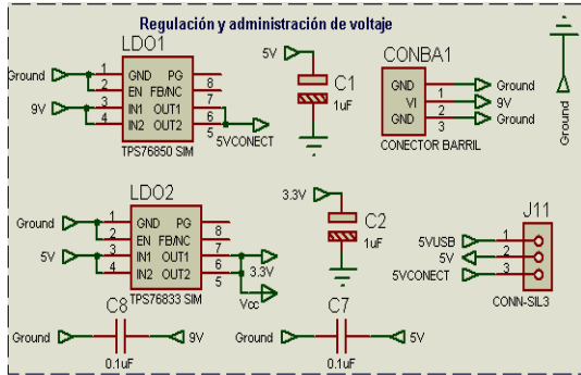
Figura 7. Regulación de voltaje.
