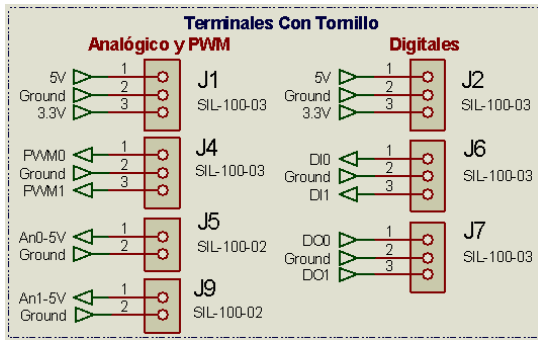
Figura 4. Terminales y conectores sensores.
